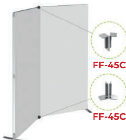
Connessione a 45°
